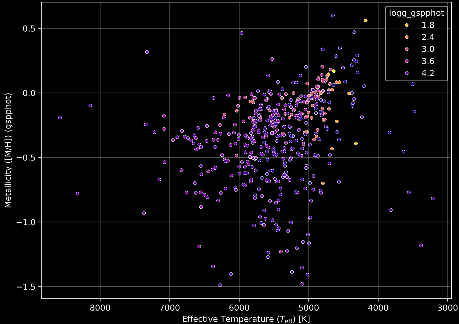
GALAH DR4 Field: [6597] Stellar Population Parameters (n= 462)
