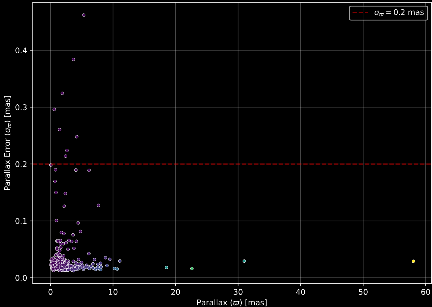
GALAH DR4 Field: [6597] Parallax Quality (n= 462)
