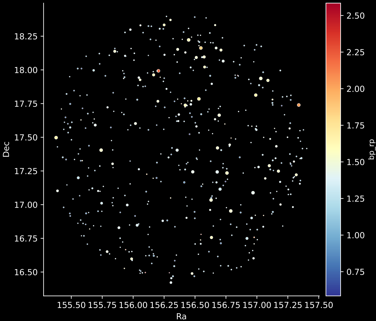
GALAH DR4 Field: [6597] Stars: 462
